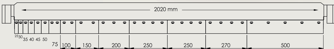
Üst Parçalı Bıçak Ölçüleri / Top Box-Pan Segmented Blade Sizes
